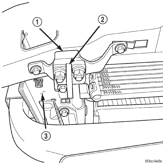
Abb. 1 Abschleppöse vorn
